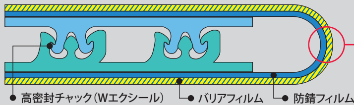
【防錆WEX袋 断面図】
