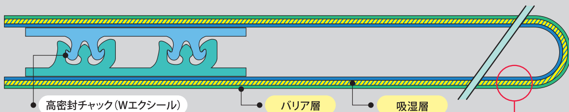
【モレキュラーシーブWエクシール袋 断面図】
