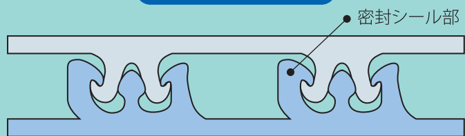
チャックの断面図
